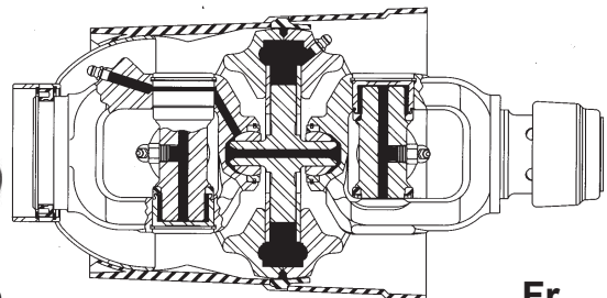
Einzigartiges Schmiersystem 4 Schmierstellen in einer Linie
