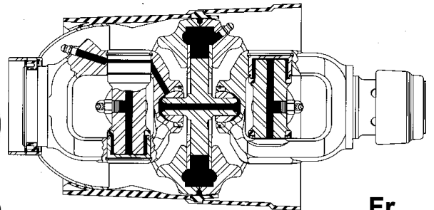
Einzigartiges Schmiersystem 4 Schmierstellen in einer Linie
